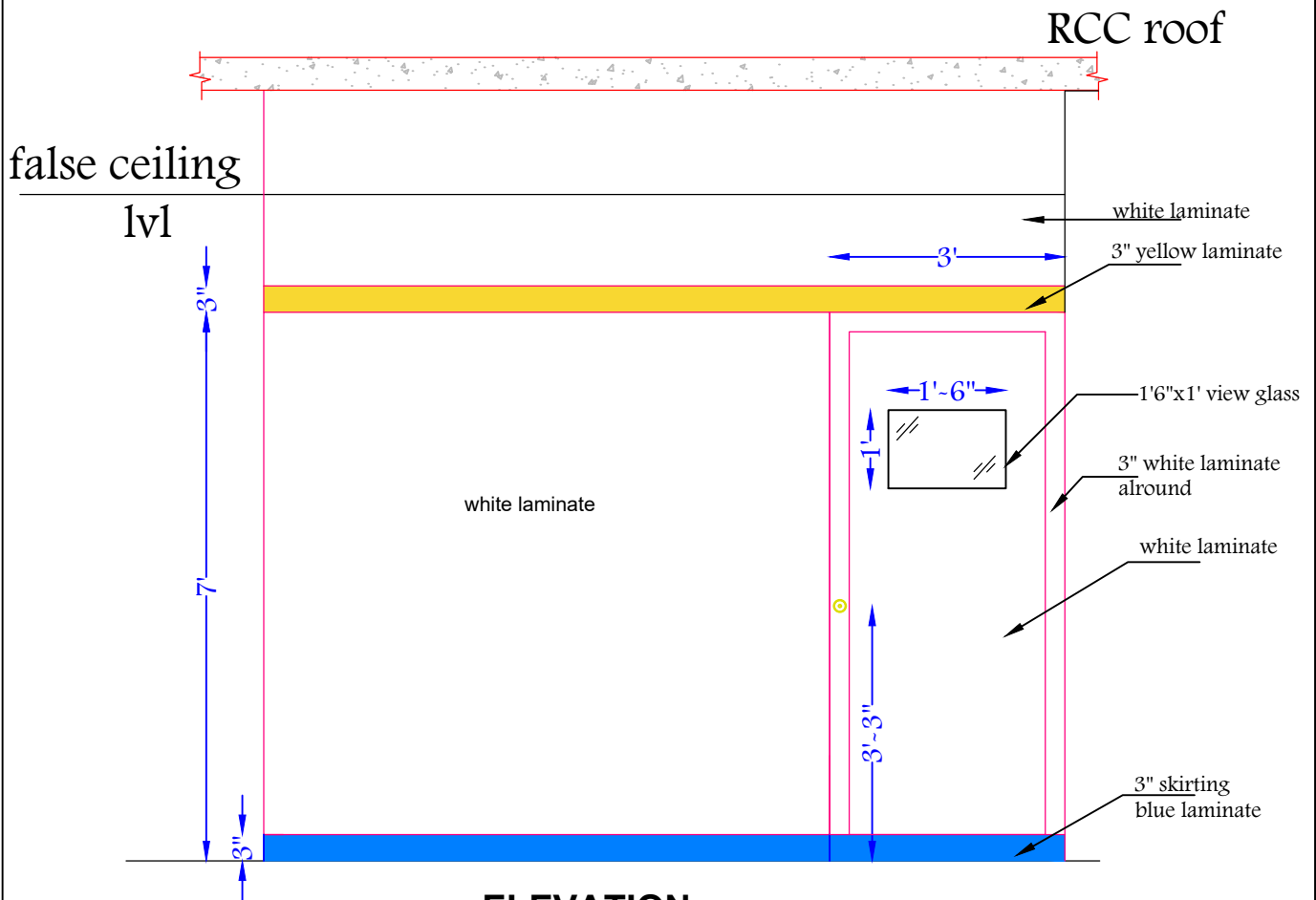
ELEVATION
